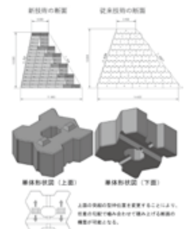
クラブブロックS型 ▶P.18
