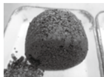
常温カンタブロ試験後の供試体（X） ▶P.9
